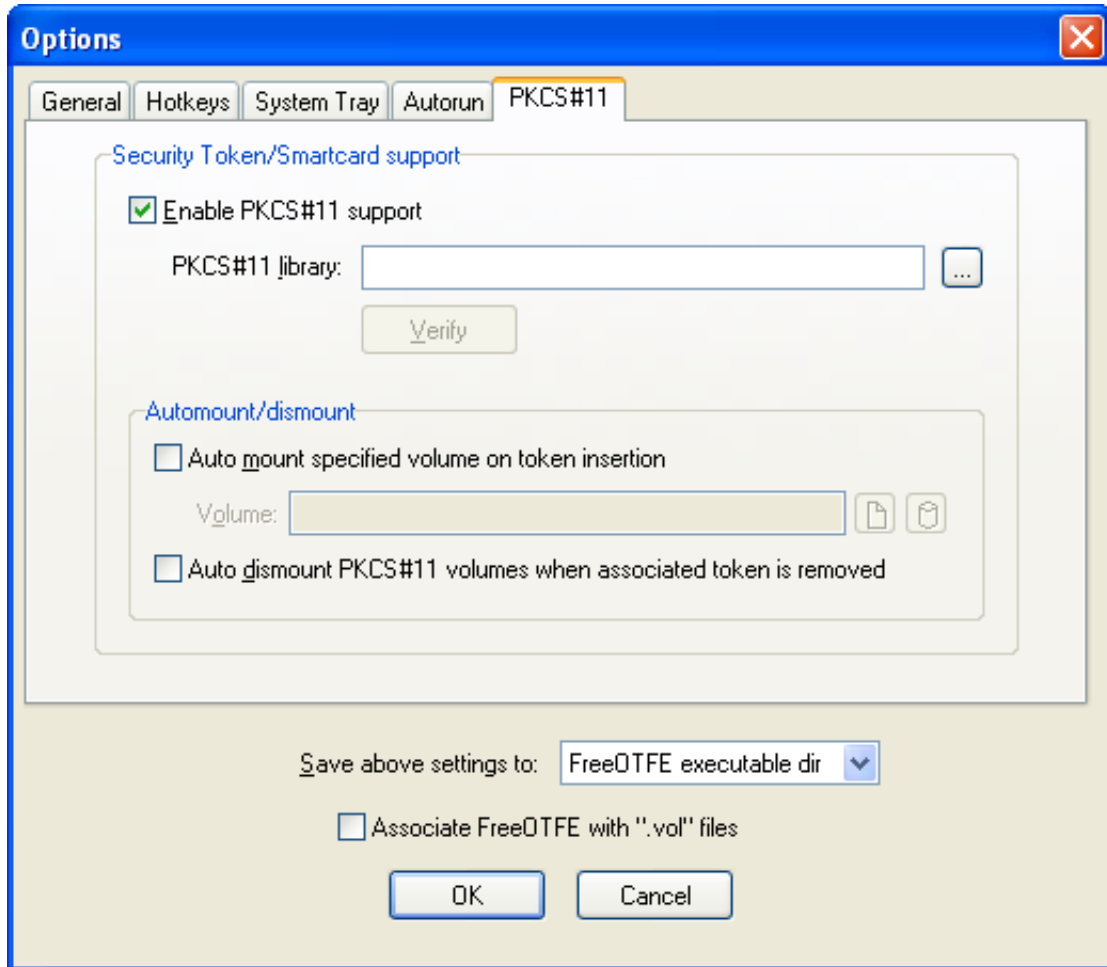
Options dialog; PKCS#11 tab
